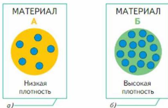
Рис. 6.1. Схема размещения молекул в материалах разной плотности
