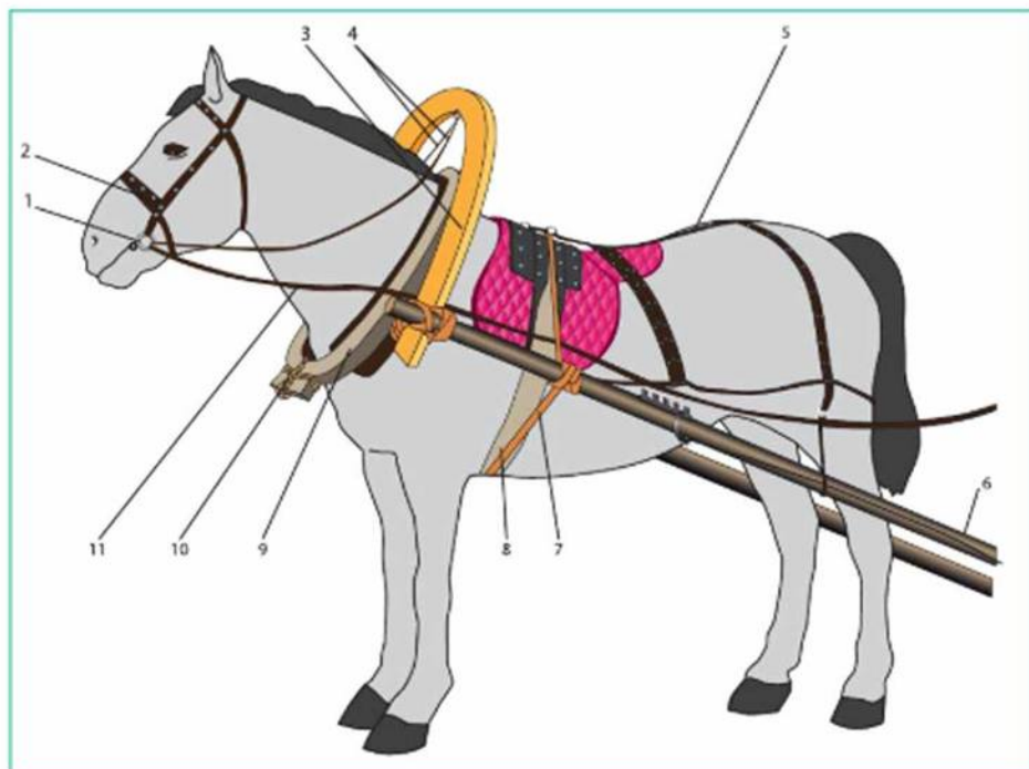
Рис. 13.6. Сбруя для оглобельно-дуговой («русской») запряжки: 1 — удила; 2 — узда; 3 — дуга; 4 — повод; 5 — шлея; 6 — оглобля; 7 — подбрюшник; 8 — подпруга; 9 — хомут; 10 — супонь; 11 — вожжи
